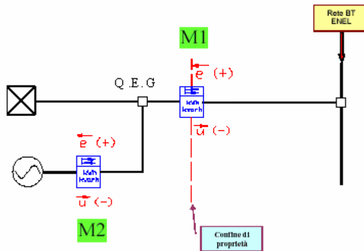
Figura 4 - Schema di collegamento dei possibili complessi di misura ENEL presso un cliente produttore.
